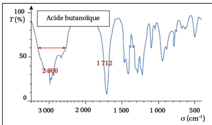
Figure 6.1 – Spectre infrarouge de l'acide butanoïque
